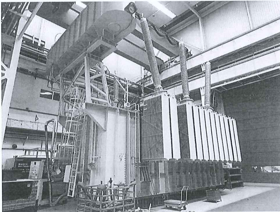
三相三绕组有载调压自耦电力变压器 OSFSZ-360000/330
