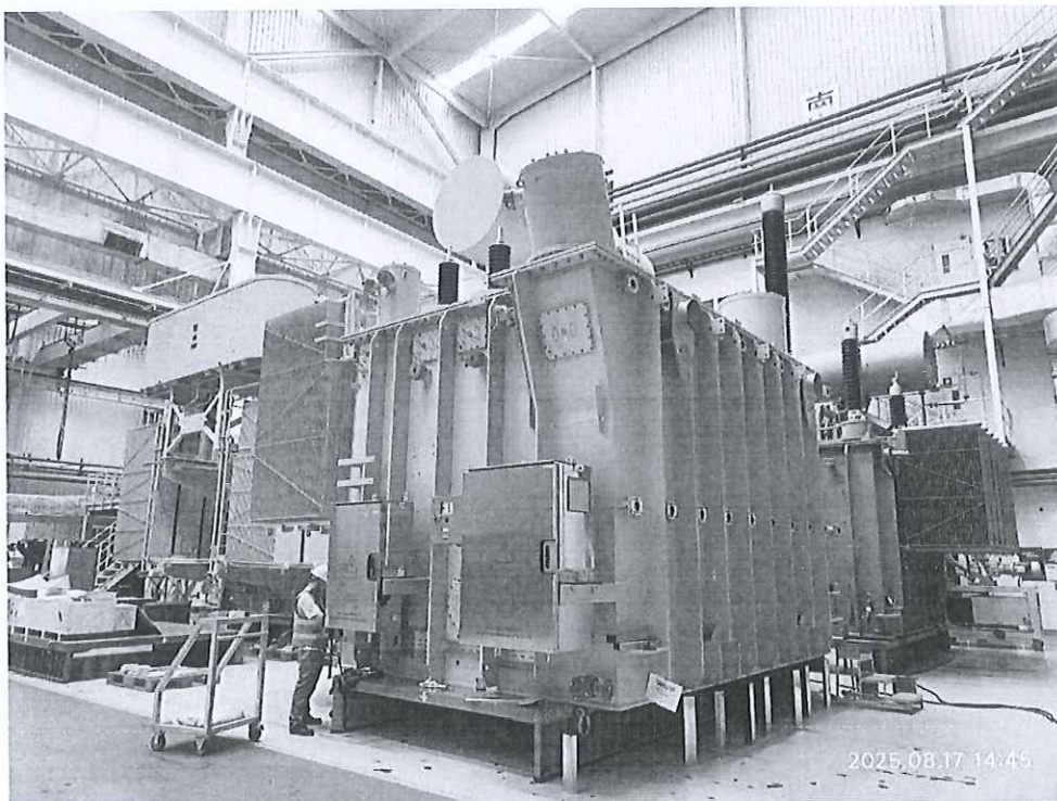
单相三绕组无励磁调压自耦电力变压器 ODFS-334000/500
