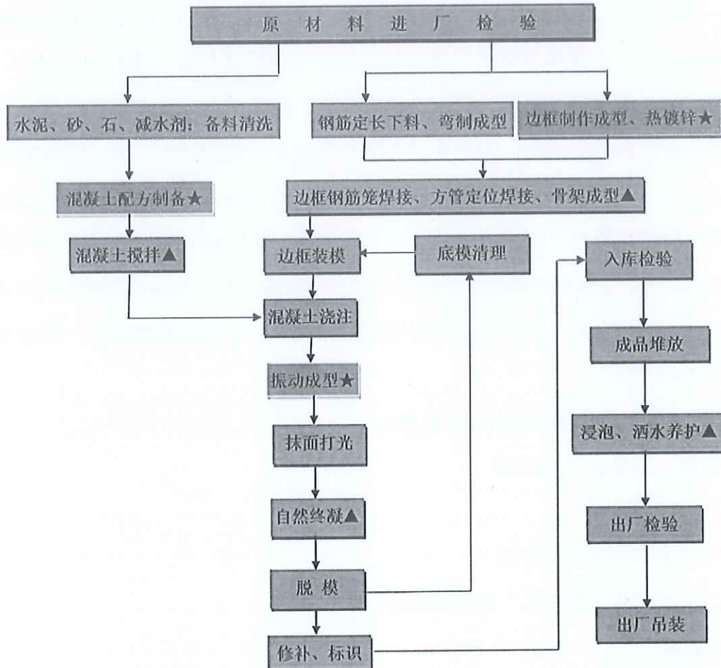
主配网混凝土电缆盖板生产工艺流程图
