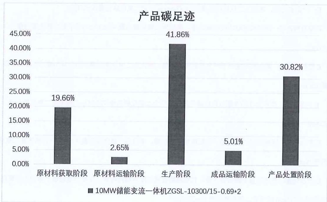
图 5.2.2 10MW 储能变流一体机 (ZGSL-10300/15-0.69*2) 生命周期阶段碳排放分布图
