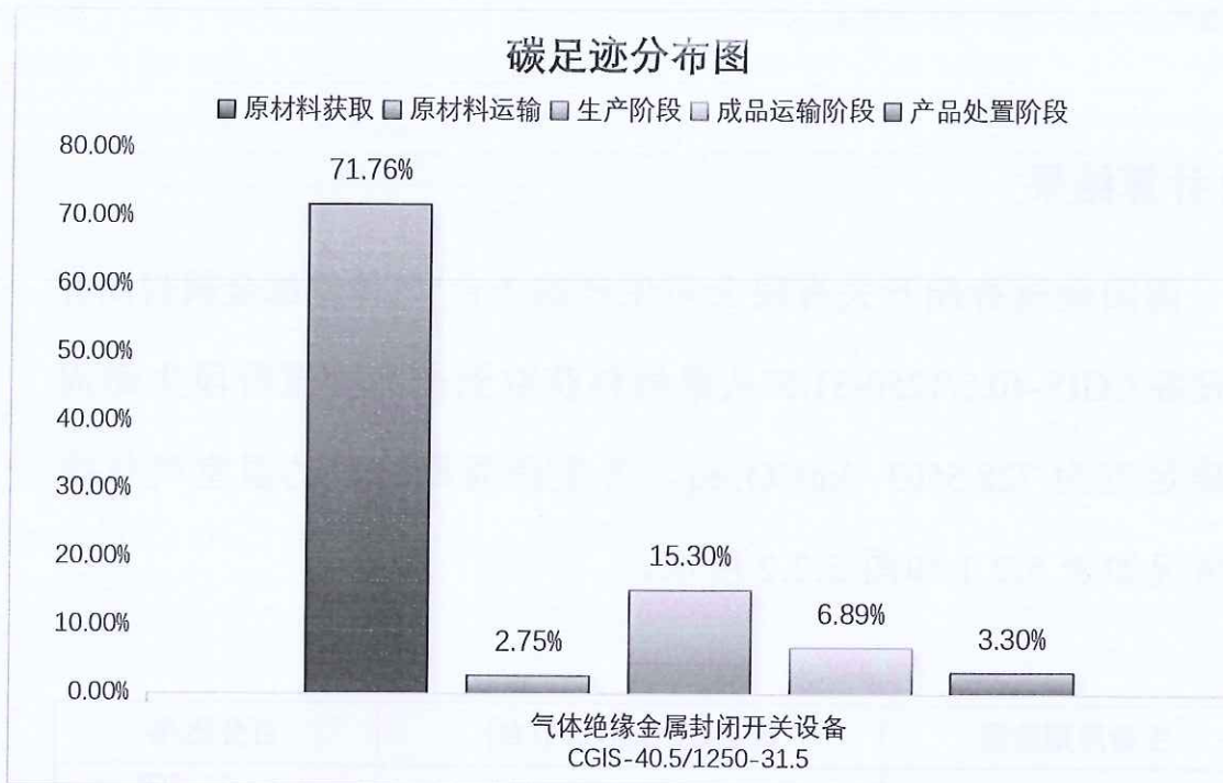
图 5.2.2 "气体绝缘金属封闭开关设备 CGIS-40.5/1250-31.5" (生命周期阶段) 碳分布图
