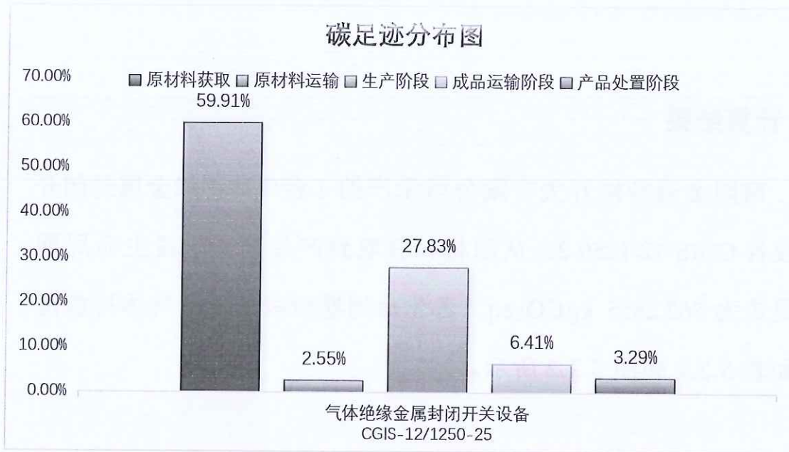
图 5.2.2 气体绝缘金属封闭开关设备 CGIS-12/1250-25 (生命周期阶段) 碳足迹分布图
