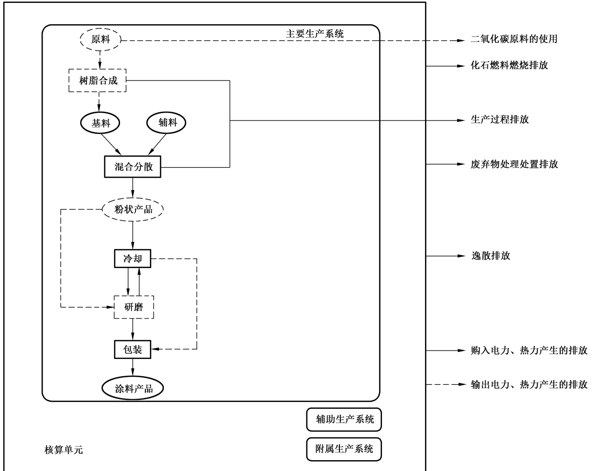
图 A.1 涂料生产企业温室气体排放及核算边界示意图
