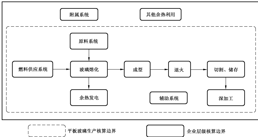
图 A.1 平板玻璃生产企业碳排放核算边界示意图
