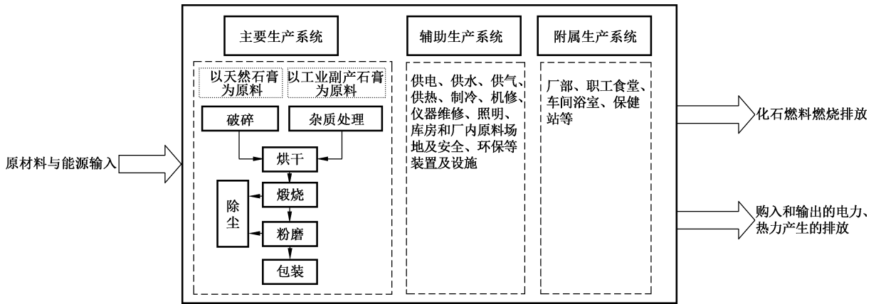
图 A.1 建筑石膏生产企业温室气体排放核算边界示意图
