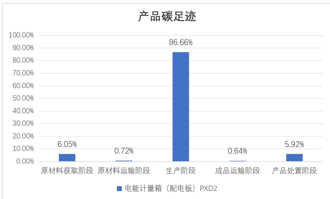
图 5.2.2 电能计量箱（配电板）（PXD2）生命周期阶段碳排放分布图
