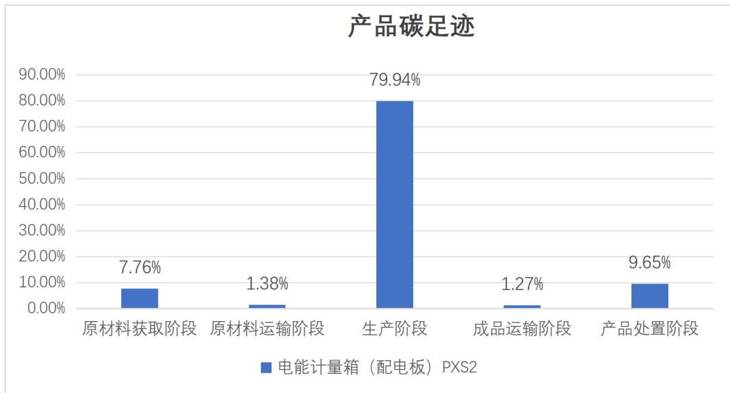
图 5.2.2 电能计量箱（配电板）（PXS2）生命周期阶段碳排放分布图
