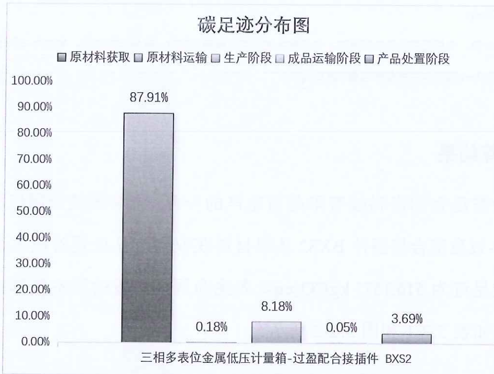
图 5.2.2 三相多表位金属低压计量箱-过盈配合接插件 BXS2 生命周期阶段碳排放分布图
