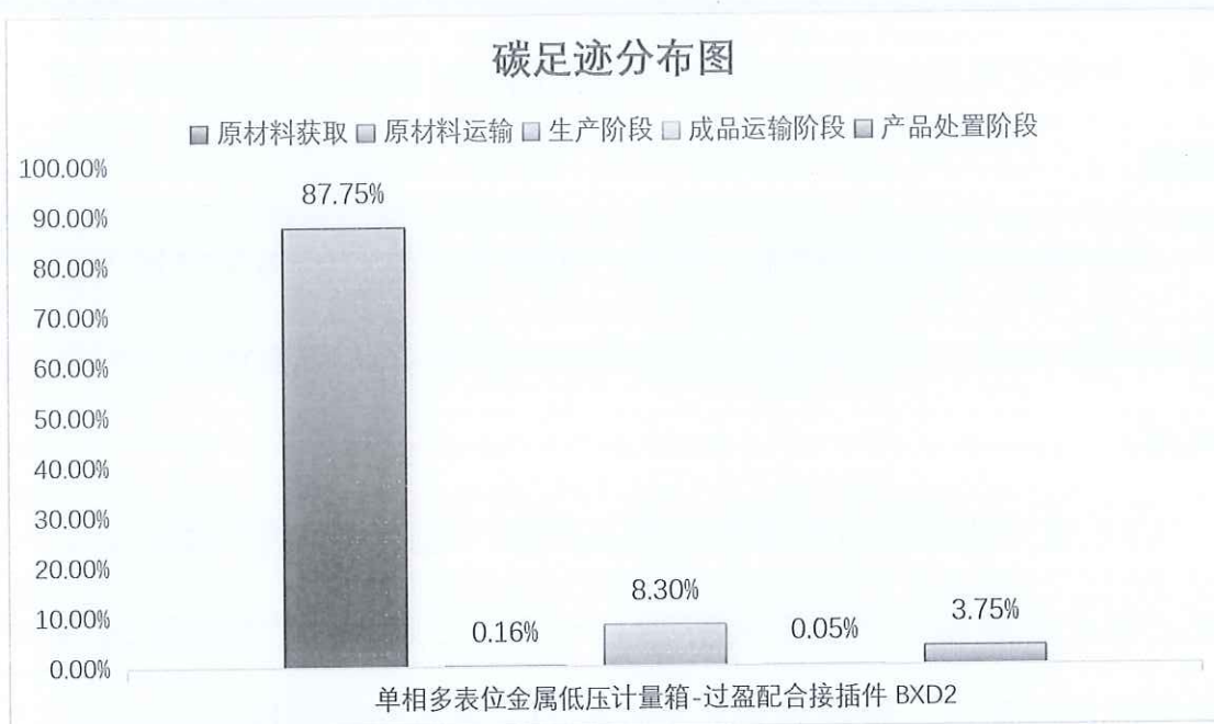
图 5.2.2 单相多表位金属低压计量箱-过盈配合接插件 BXD2 (生命周期阶段碳排放分布图)
