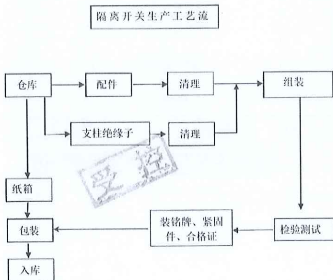
生产工艺流程图
