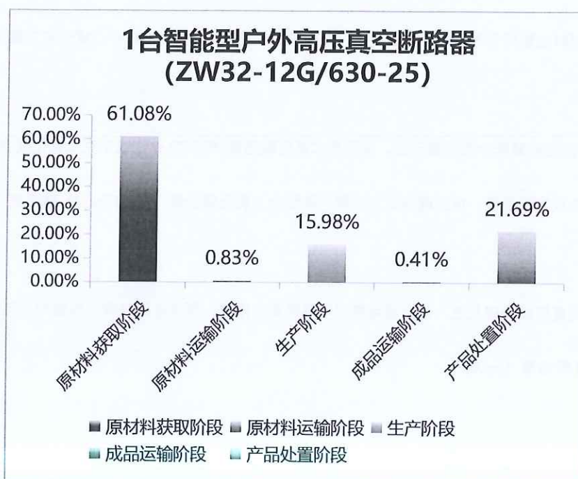
图 5.2-2 1 台智能型户外高压真空断路器 (ZW32-12G/630-25)
