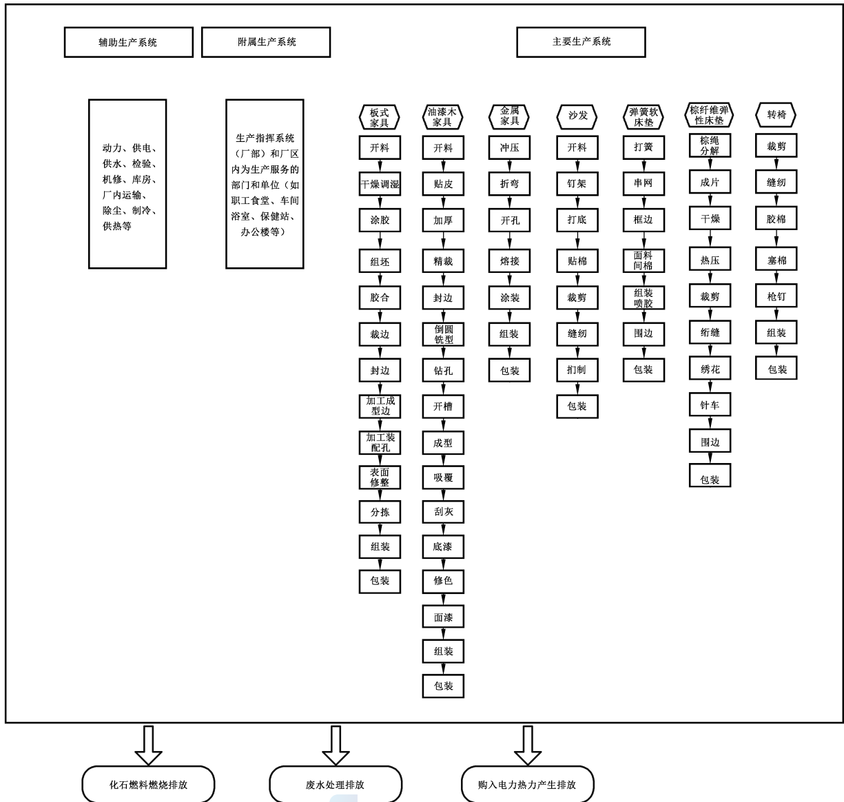
图 A.1 典型家具生产企业温室气体核算边界示意图
