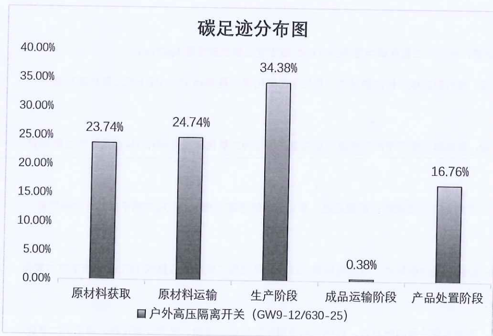
图 5.2.1.2 户外高压隔离开关 (GW9-12/630-25) 生命周期阶段碳排放分布图
