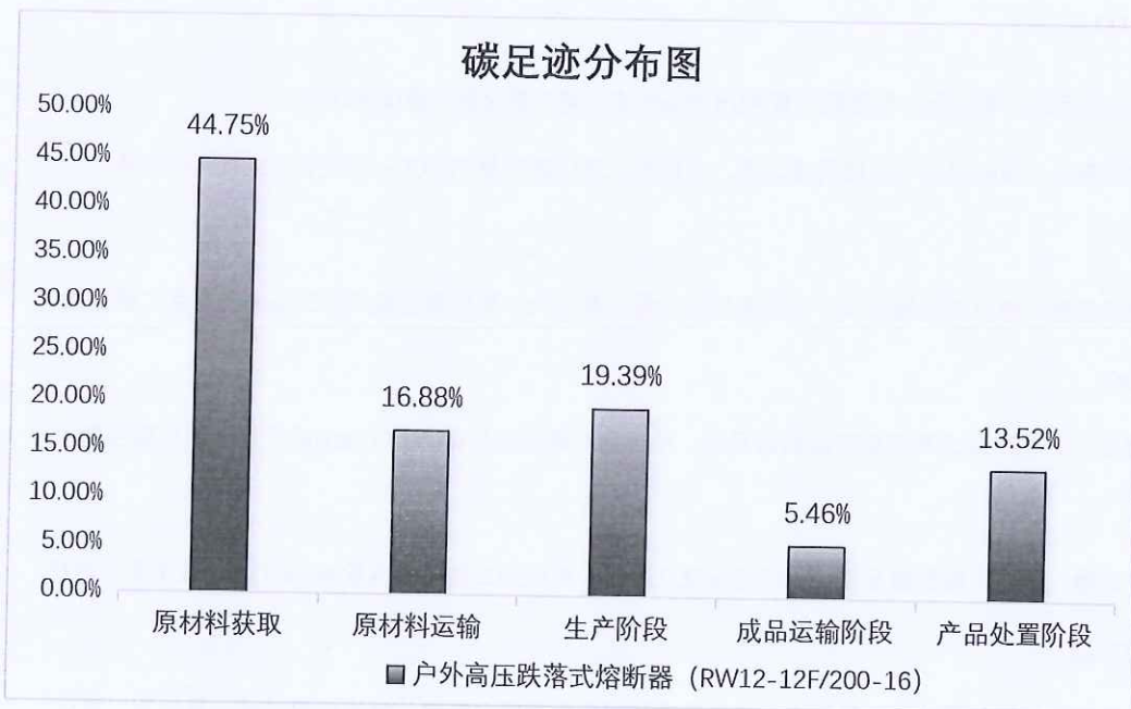
图 5.2.1.2 户外高压跌落式熔断器 (RW12-12F/200-16) 生命周期阶段碳排放分布图
