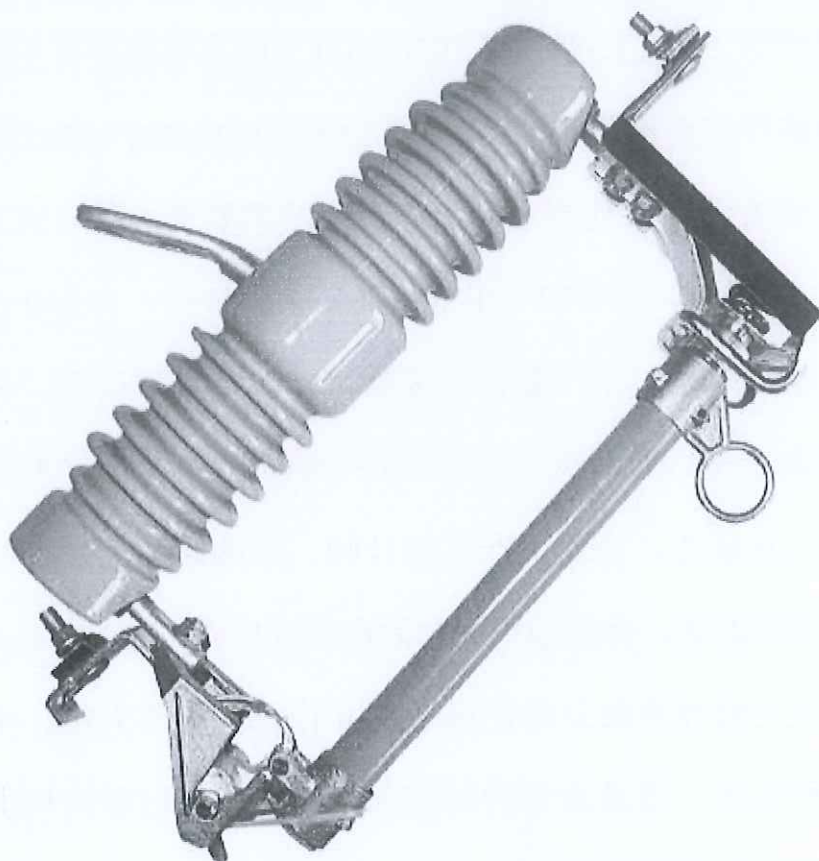
户外高压跌落式熔断器 (RW12-12F/200-16)
