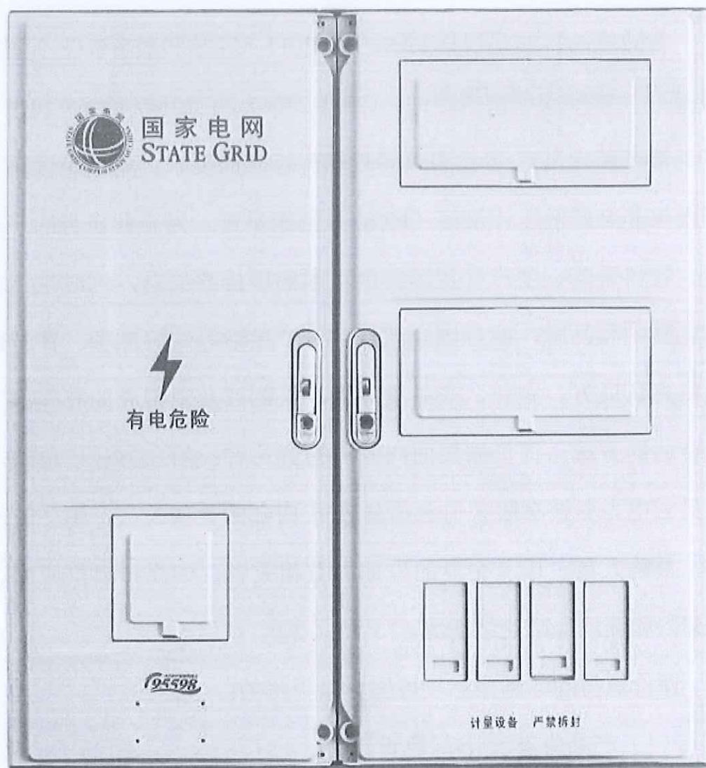
三相多表位非金属低压计量箱（PXS2）
