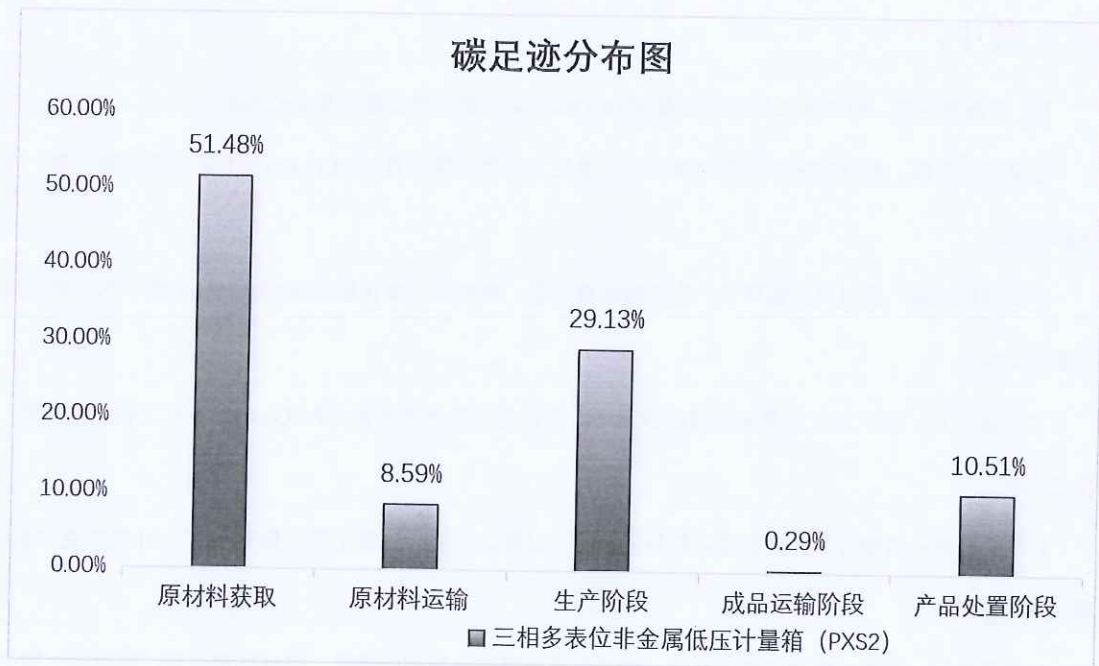
图 5.2.1.2 三相多表位非金属低压计量箱 (PXS2) 生命周期阶段碳排放分布图
