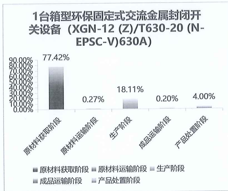
图 5.2-2 1 台箱型环保固定式交流金属封闭开关设备 (XGN-12 (Z)/T630-20 (N-EPSC-V)630A)
