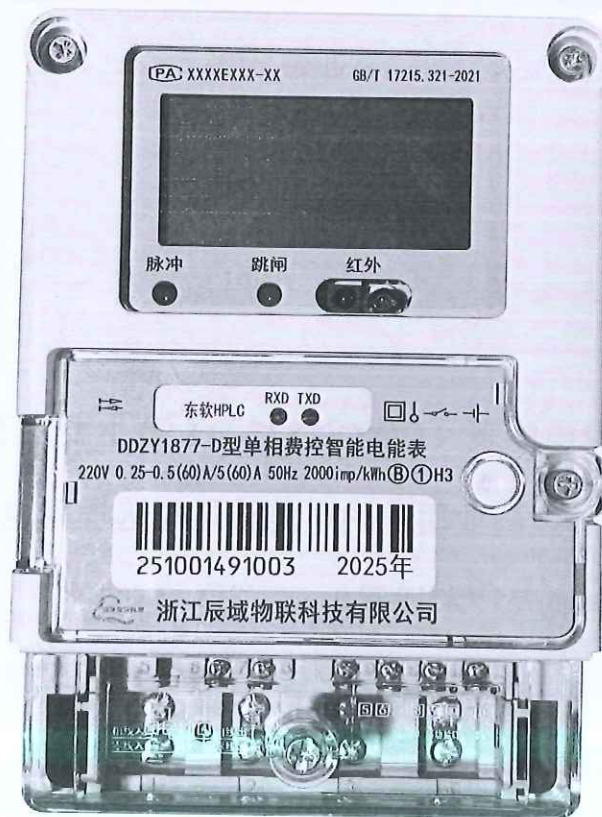
单相费控智能电能表（DDZY1877-D）
