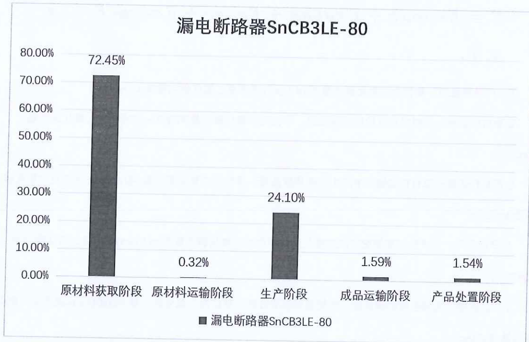
图 5.2.2 漏电断路器 (SnCB3LE-80) 生命周期阶段碳排放分布图
