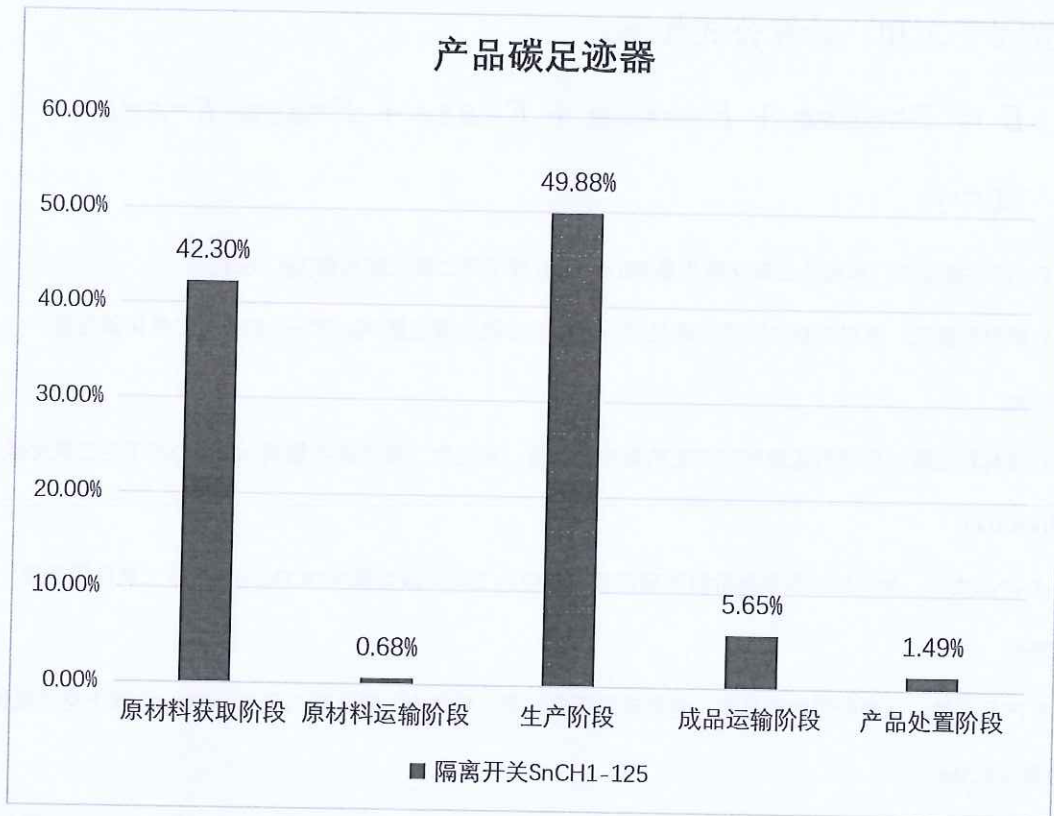
图 5.2.2 隔离开关 (SnCH1-125) 生命周期阶段碳排放分布图
