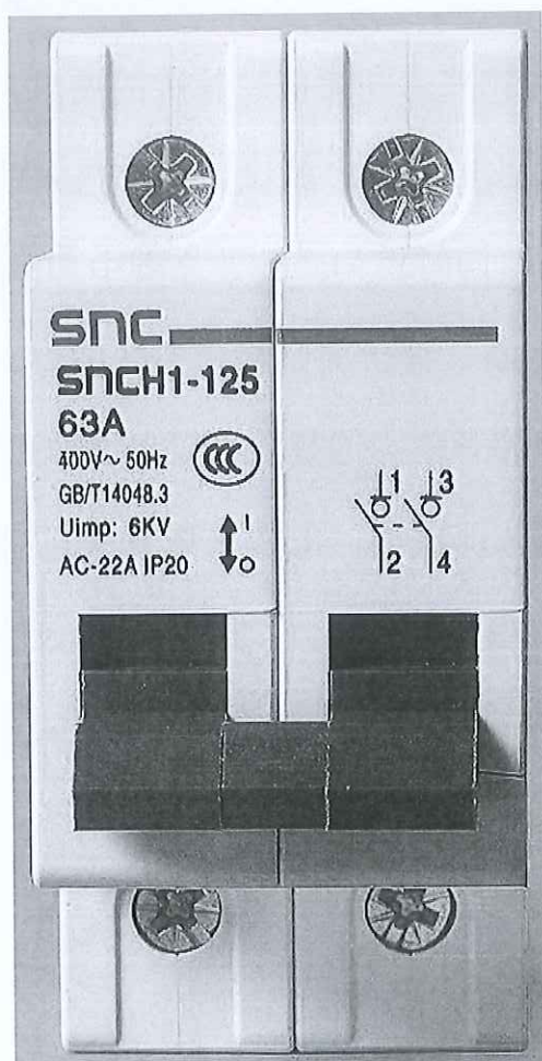
隔离开关 (SnCH1-125)
