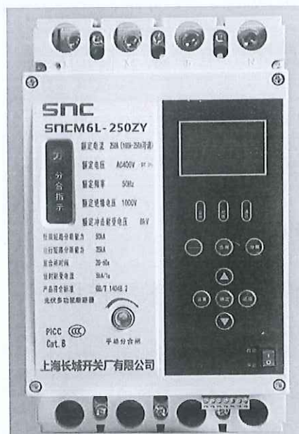
剩余电流动作断路器（SnCM6L-250ZY）
