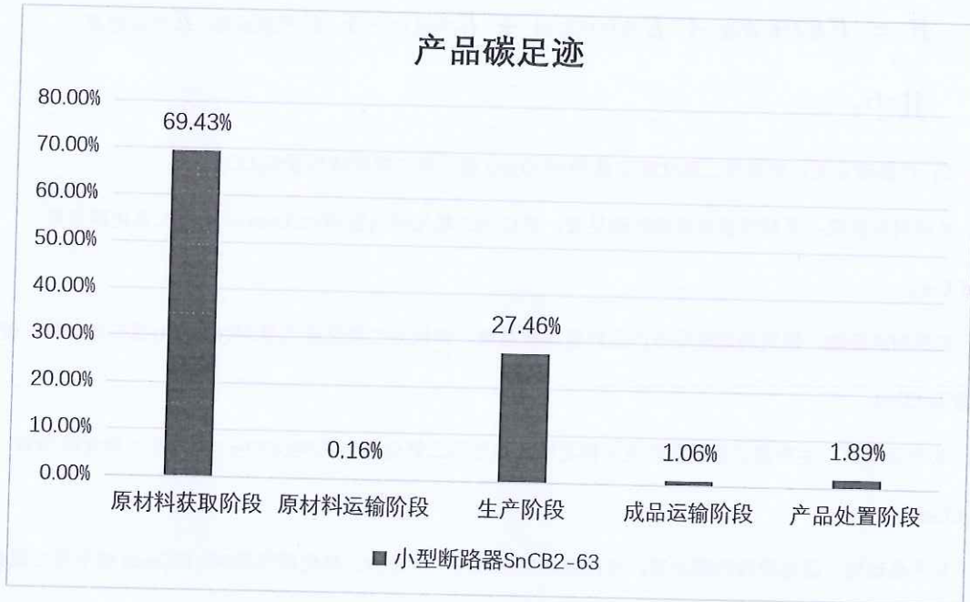
图 5.2.2 小型断路器 (SnCB2-63) 生命周期阶段碳排放分布图
