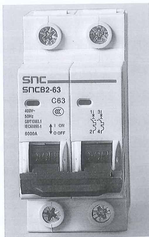
小型断路器 (SnCB2-63)
