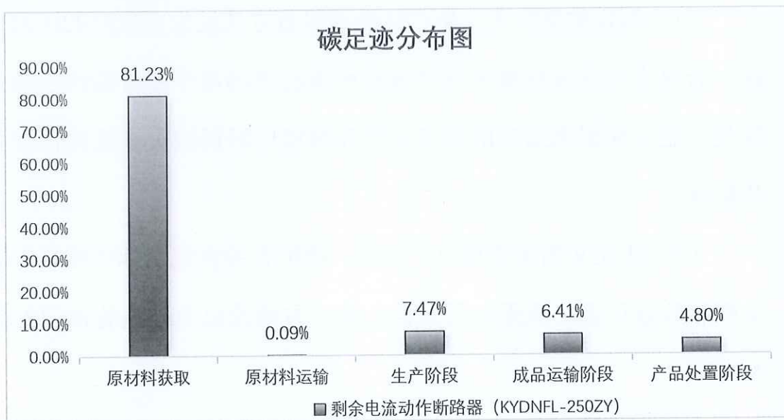
图 5.2.1.2 剩余电流动作断路器 (KYDNFL-250ZY) 生命周期阶段碳排放分布图
