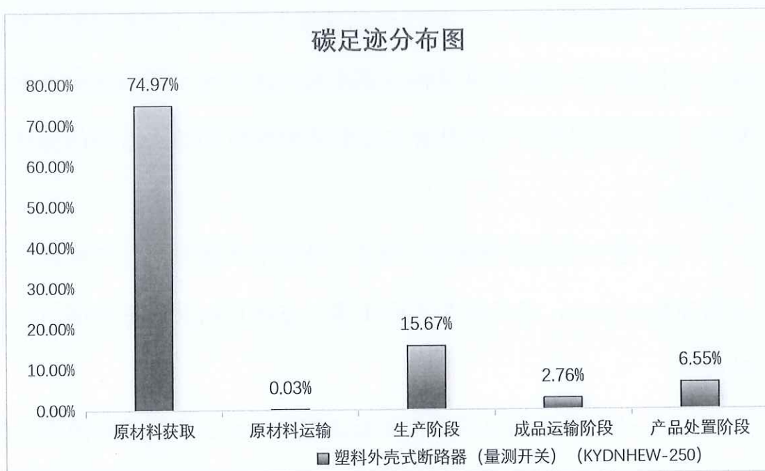
图 5.2.1.2 塑料外壳式断路器（量测开关）（KYDNHEW-250）生命周期阶段碳排放分布图
