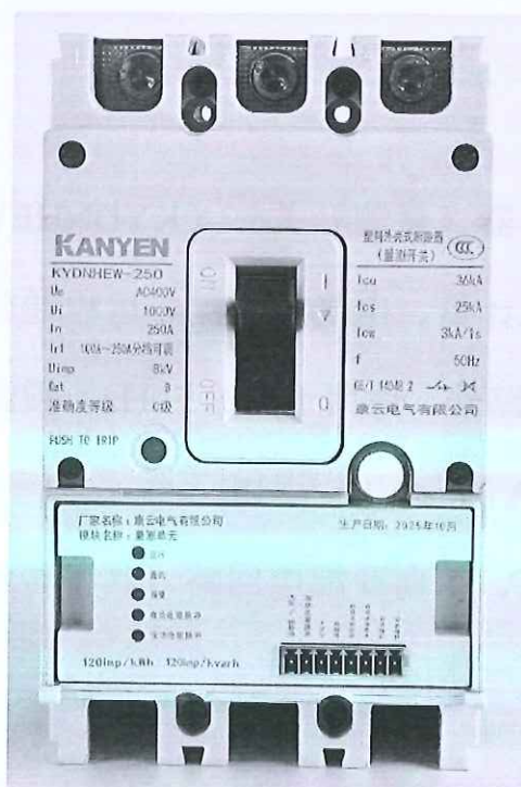
塑料外壳式断路器（量测开关）（KYDNHEW-250）
