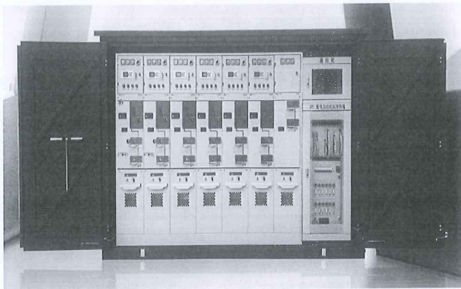
预装式金属封闭环网箱（JKHWX-12）
