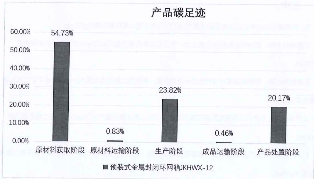
图 5.2.2 预装式金属封闭环网箱（JKHWX-12）生命周期阶段碳排放分布图
