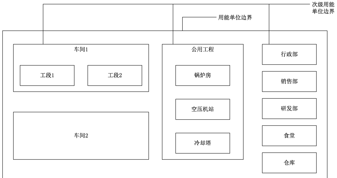
图 1 企业耗能边界示意图
