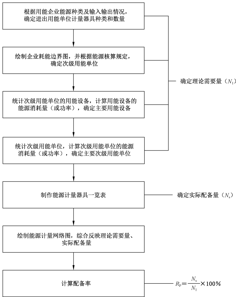
图 2 企业能源计量器具配备率检查流程
