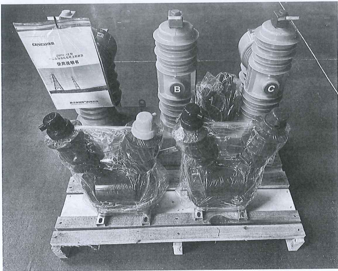
一二次融合成套柱上断路器（ZW32-12/630-25）
