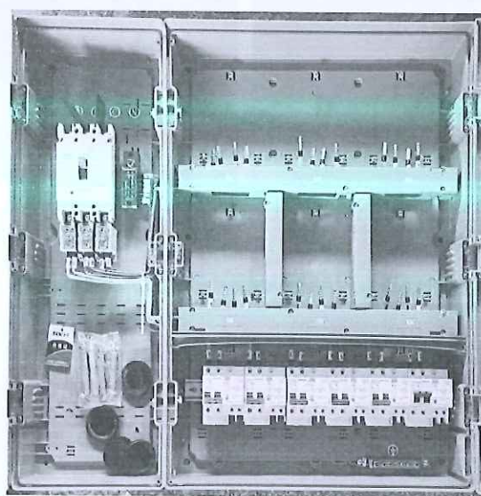
电能计量箱（配电板）(PC+ABS) (PXD2)
