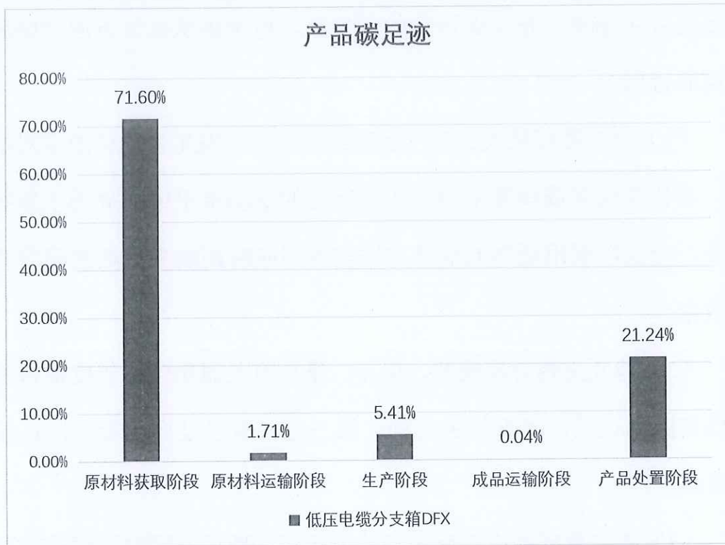
图 5.2.2 低压电缆分支箱（DFX）生命周期阶段碳排放分布图
