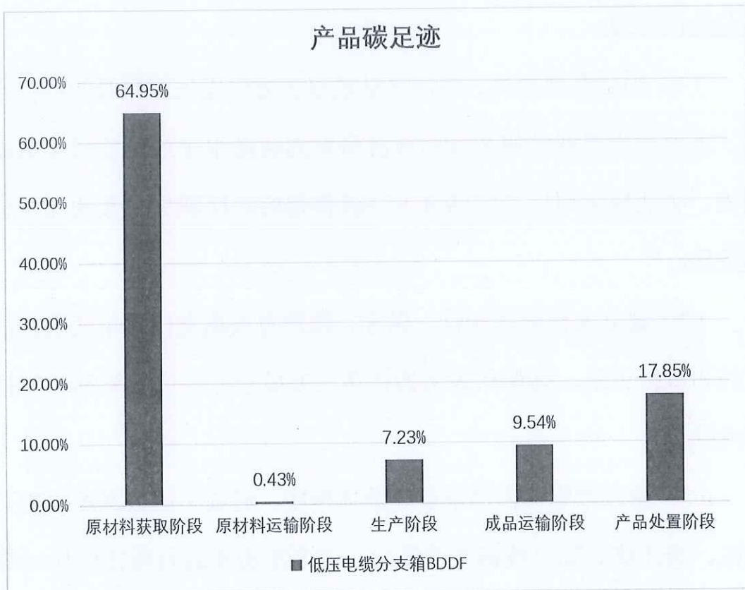
图 5.2.2 低压电缆分支箱（BDDF）生命周期阶段碳排放分布图
