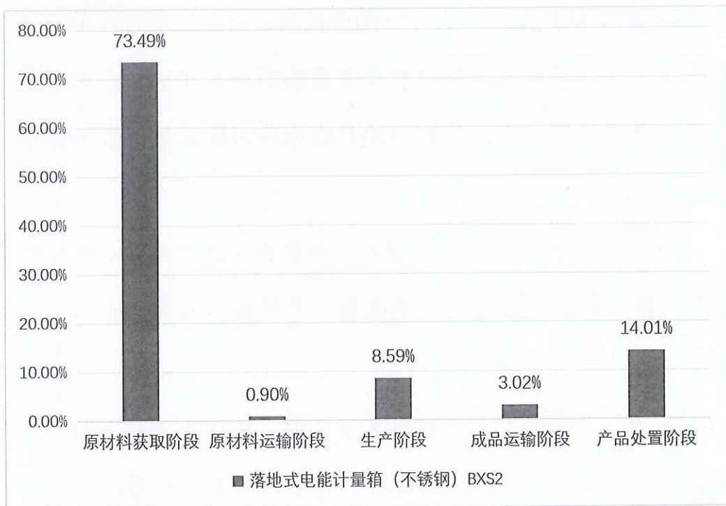
图 5.2.2 落地式电能计量箱（不锈钢）（BXS2）生命周期阶段碳排放分布图
