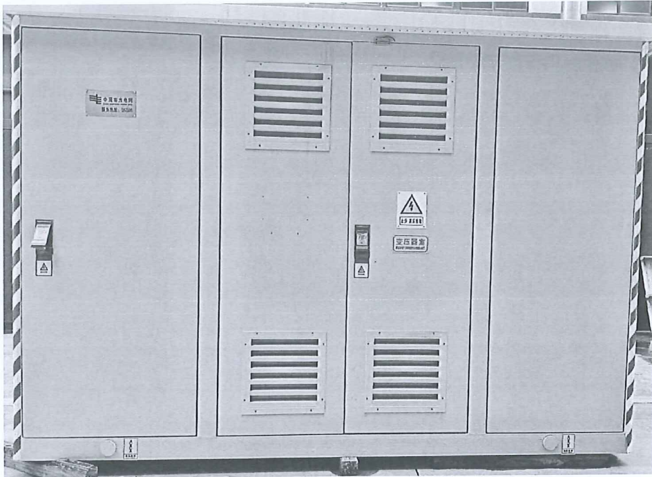
箱式变电站（YB□-12/0.4-1600）
