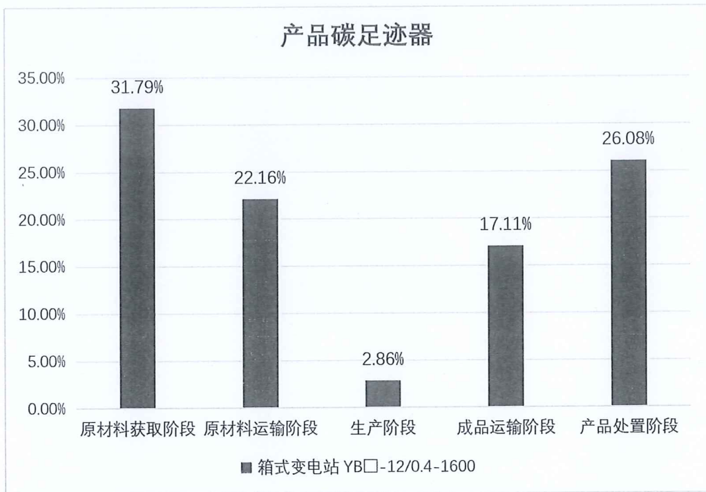
图 5.2.2 箱式变电站（YB□-12/0.4-1600）生命周期阶段碳排放分布图
