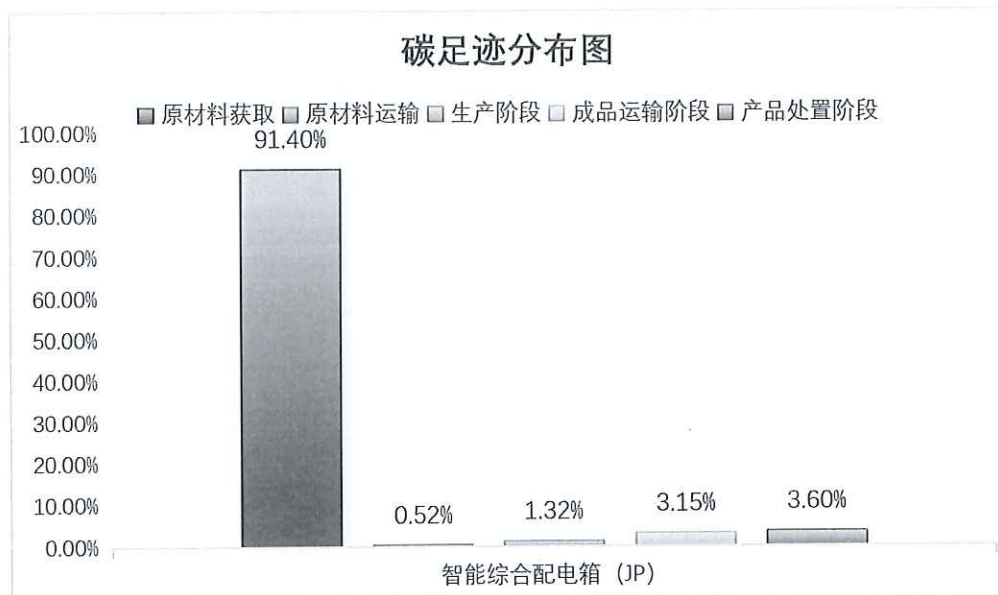
图 5.2-2 综合配电箱生命周期阶段碳排放分布图
