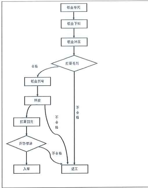
钣金制作流程图：
