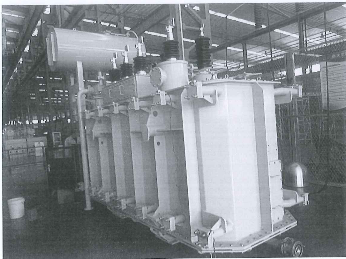
电力变压器 SZ22-31500/35-NX1 31500kVA
