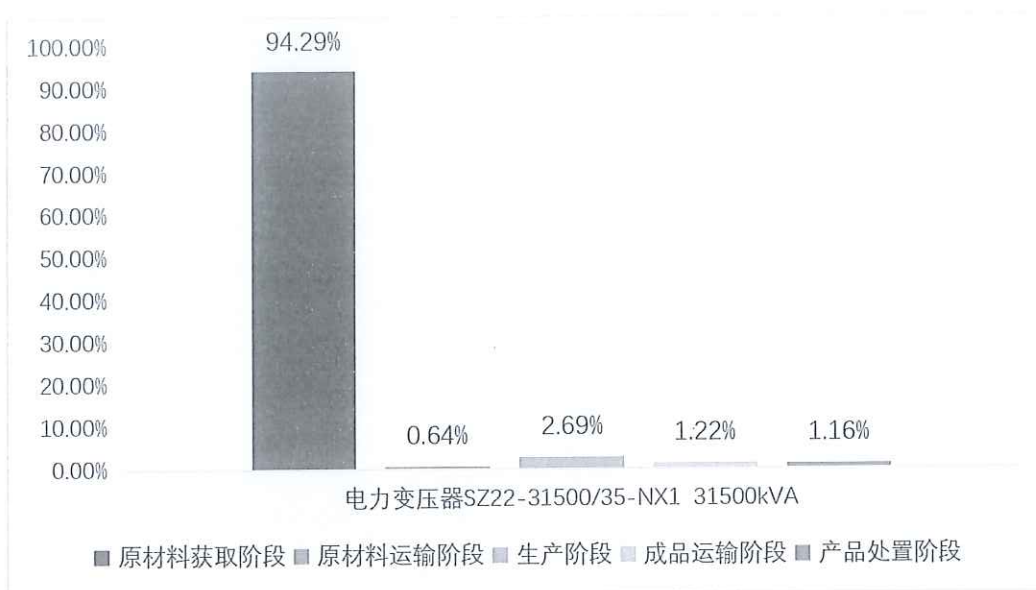
图 5.2-1 电力变压器 SZ22-31500/35-NX1 31500kVA 生命周期阶段碳排放分布图
