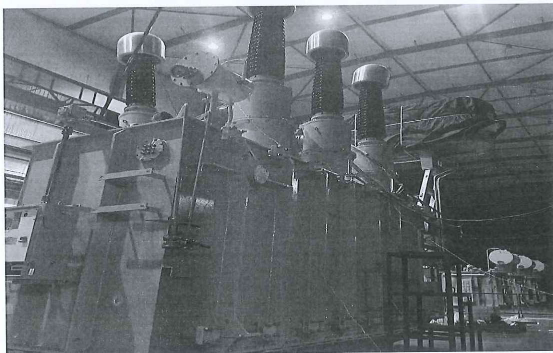
电力变压器 SZ22-31500/35-NX1 31500kVA
