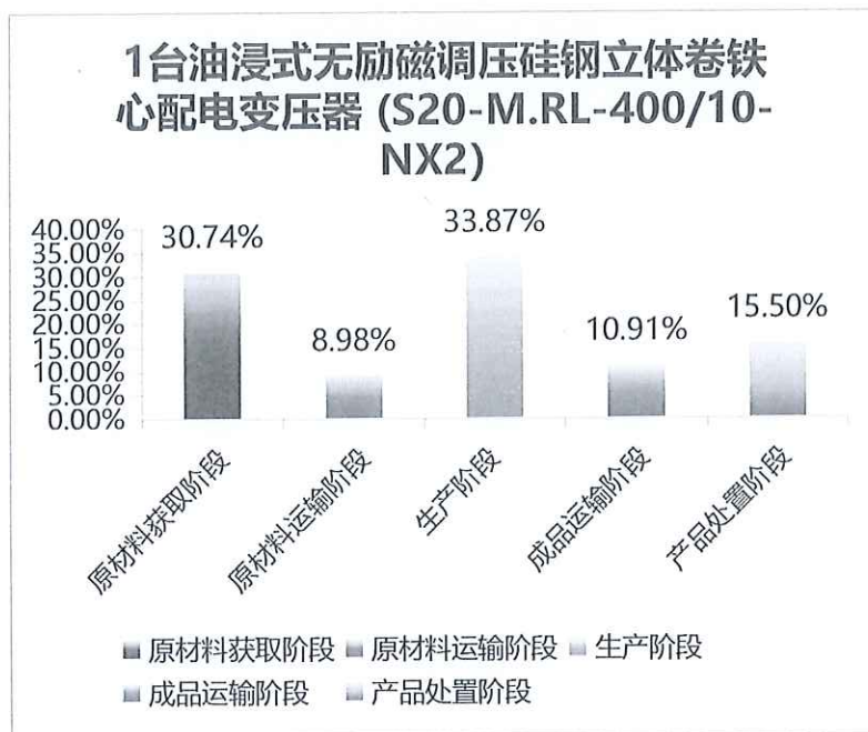
图 5.2-2 一台油浸式无励磁调压硅钢立体卷铁心配电变压器 (S20-M.RL-400/10-NX2) 生命周期阶段碳排放分布图
