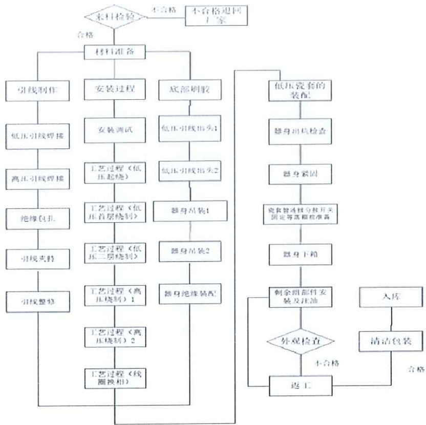
变压器装配工艺流程图
