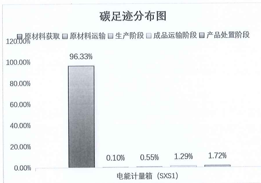
图 5.2.7-2 产品生命周期阶段碳排放分布图
