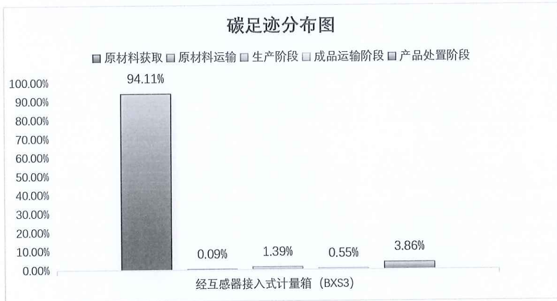
图 5.2.4-2 产品生命周期阶段碳排放分布图
