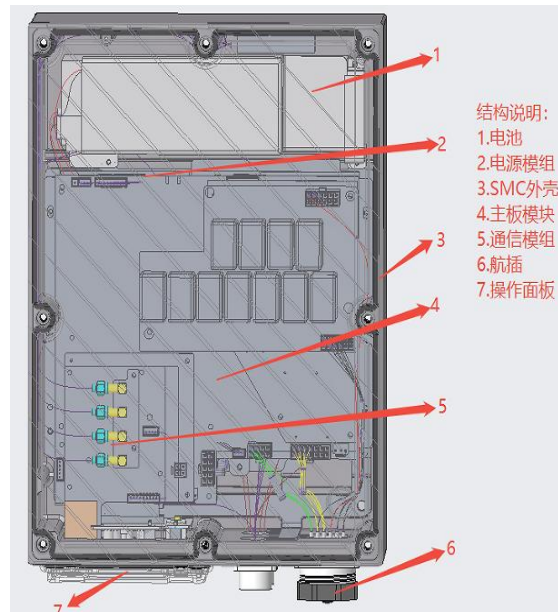
配电自动化馈线终端 KD-100FDG03L
