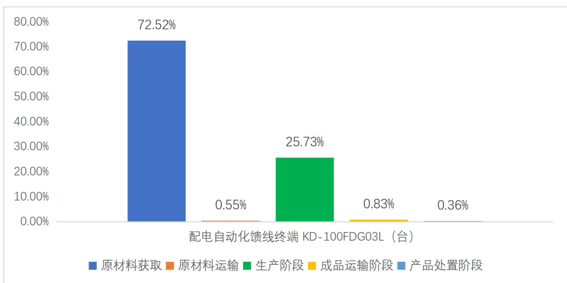
图 5.2.2 配电自动化馈线终端（KD-100FDG03L）生命周期阶段碳排放分布图
