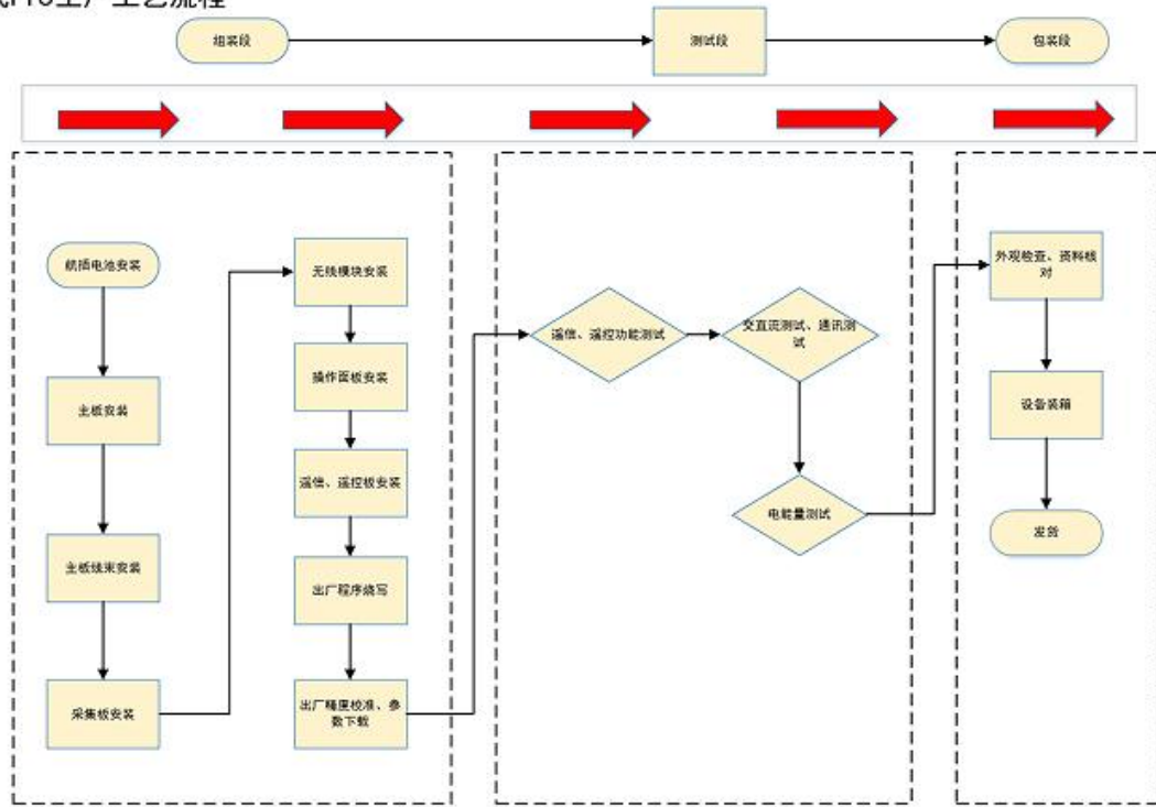
箱式FTU生产工艺流程
