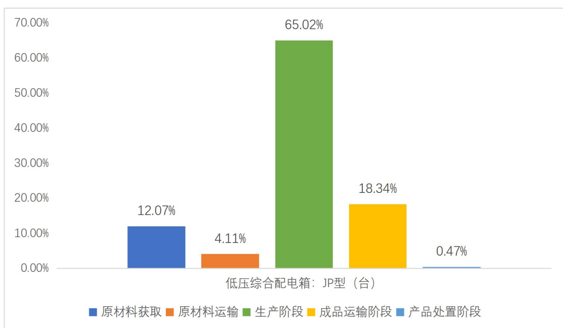
图 5.2.2 低压综合配电箱：JP 型生命周期阶段碳排放分布图
