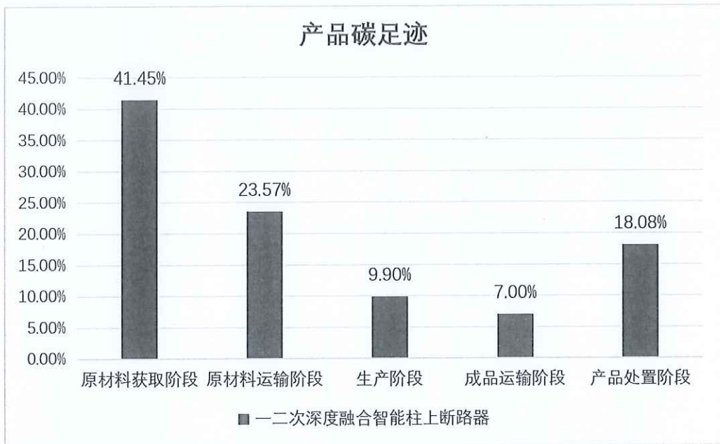
图 5.2.2 一二次深度融合智能柱上断路器 (ZW32-12/630-20) 生命周期阶段碳排放分布图
