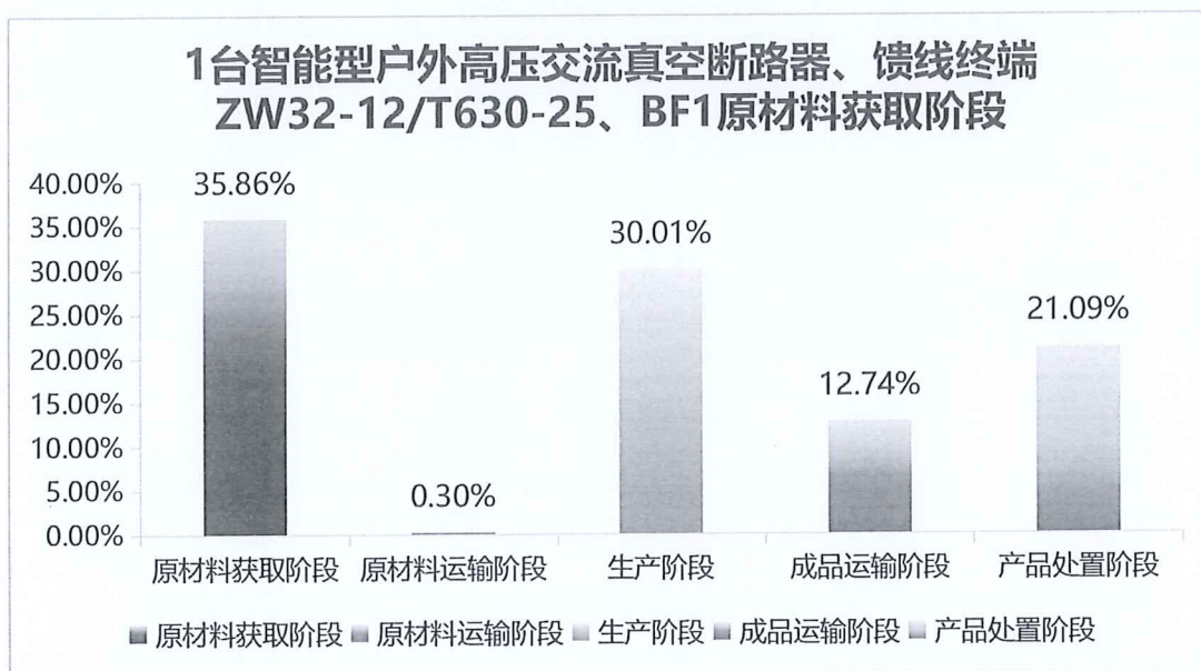
图 5.2-2 一台智能型户外高压交流真空断路器、馈线终端（ZW32-12/T630-25、BF1）生命周期阶段碳排放分布图
