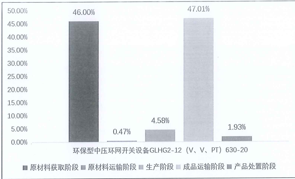
图 5.2-2-3 1 台 环保型中压环网开关设备 GLHG2-12 (V、V、PT)/630-20 生命周期阶段碳排放分布图
