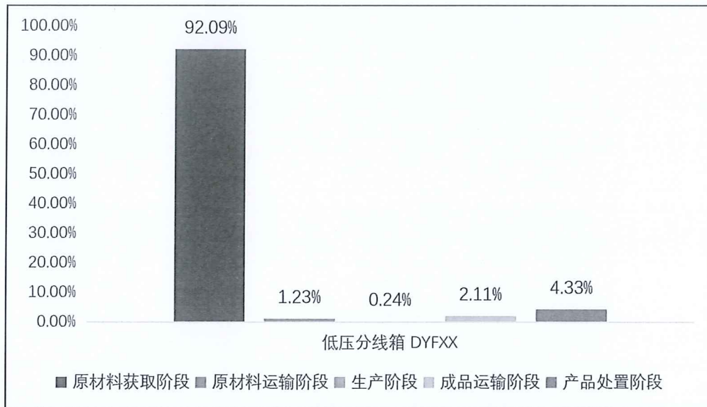
图 5.2-2-1 1 台 低压分线箱 DYFXX 生命周期阶段碳排放分布图
