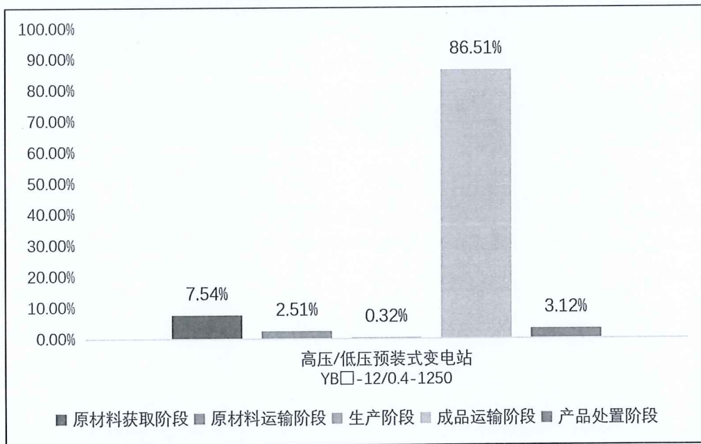
图 5.2-2-5 1 台 高压 / 低压预装式变电站 YB□-12/0.4-1250 生命周期阶段碳排放分布图
