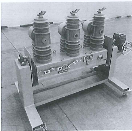
一二次融合标准化柱上真空断路器 GLZW32-12/630-25
