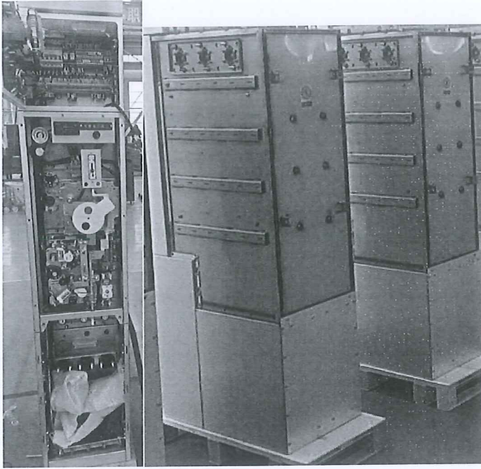
环保型中压环网开关设备 GLHG2-12 (V、V、PT)/630-20
