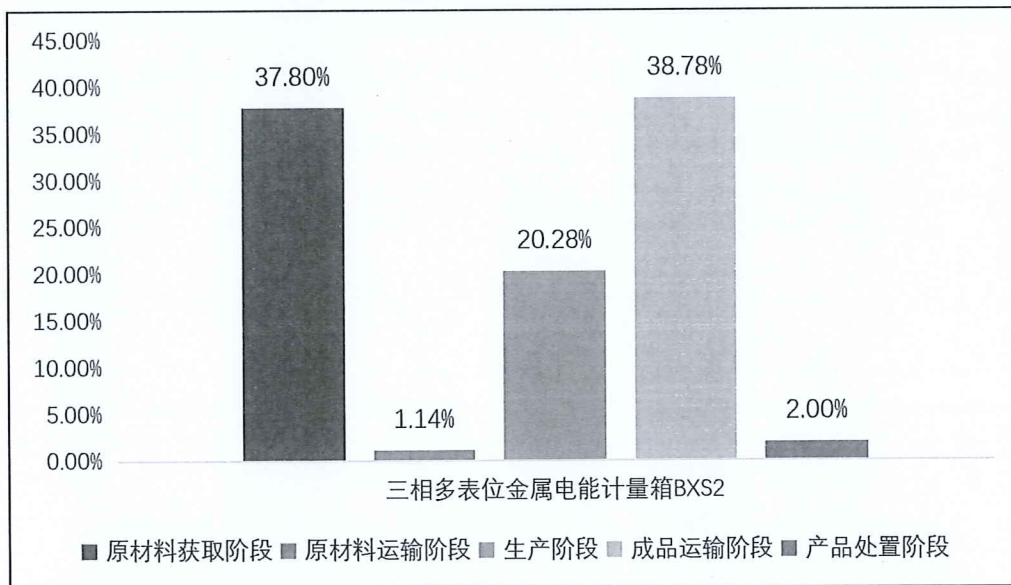
图 5.2-2-4 1 台三相多表位金属电能计量箱 BXS2 生命周期阶段碳排放分布图
