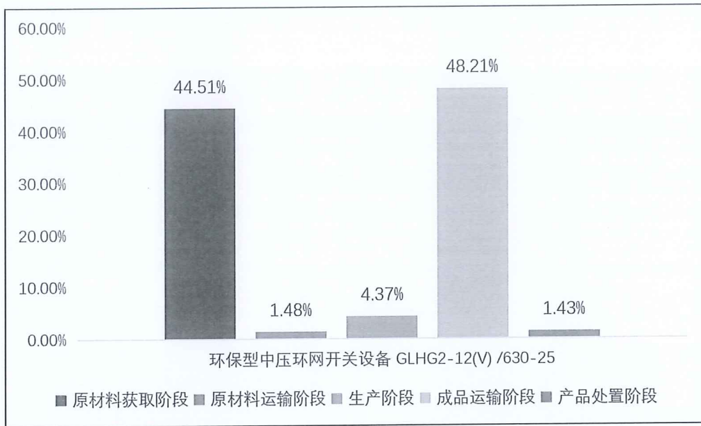
图 5.2-2-2 1 台 环保型中压环网开关设备 GLHG2-12 (V)/630-25 生命周期阶段碳排放分布图
