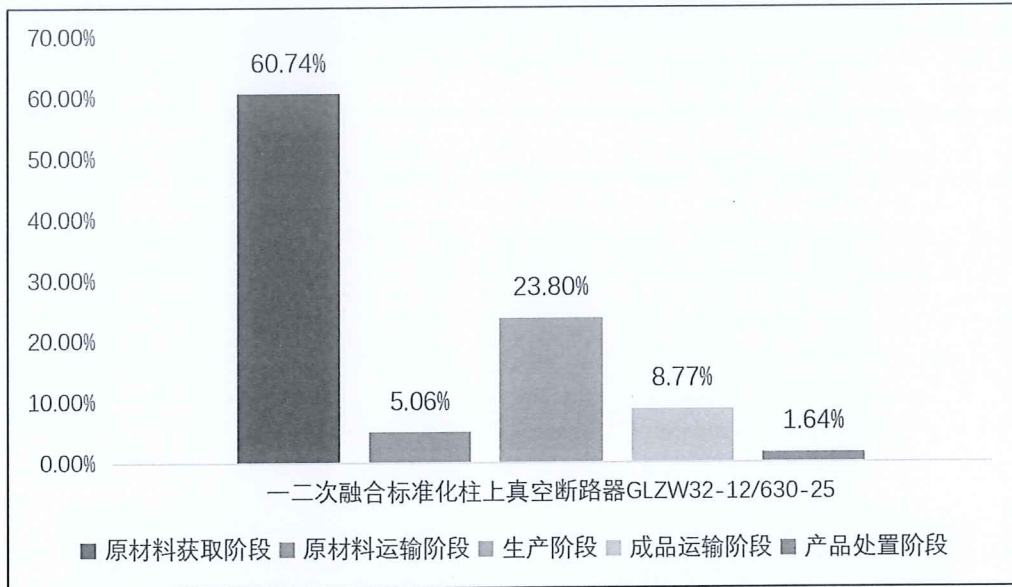
图 5.2-2-6 1 台 一二次融合标准化柱上真空断路器 GLZW32-12/630-25 生命周期阶段碳排放分布图
