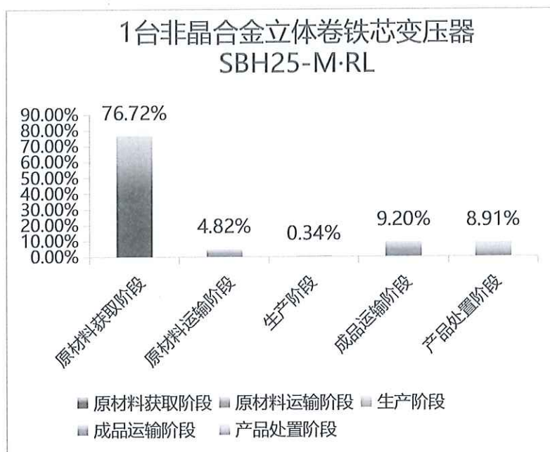
图 5.2-2 一台非晶合金立体卷铁芯变压器（SBH25-M·RL）生命周期阶段碳排放分布图
