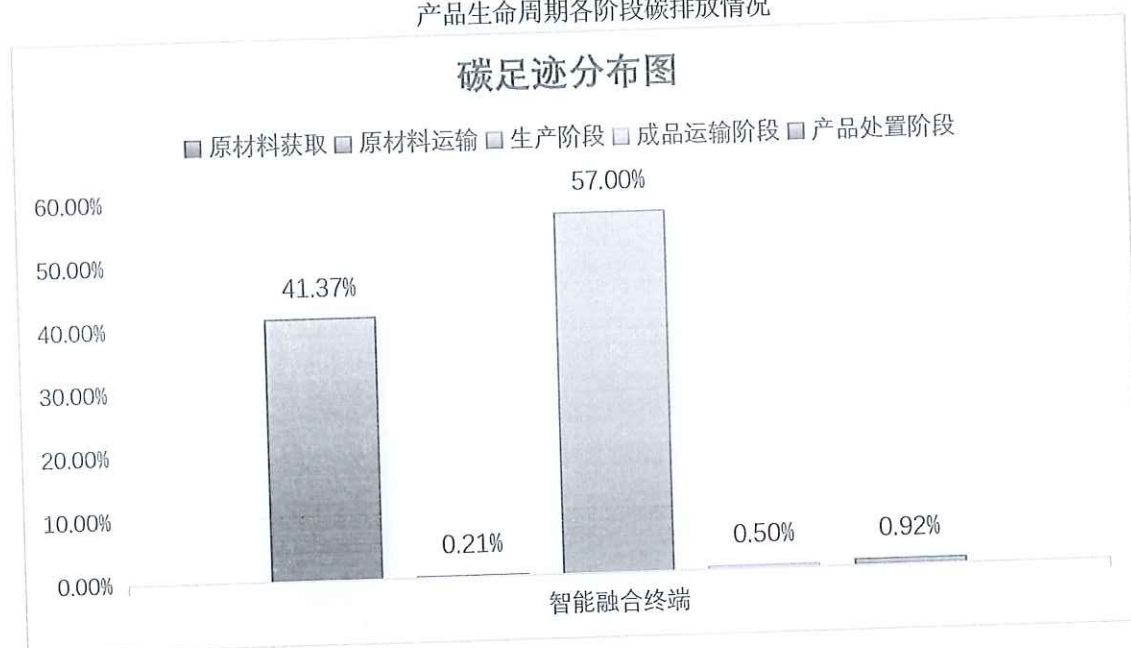
图 5.2-2 1 台智能综合配电箱（JP） 产品生命周期阶段碳排放分布图
