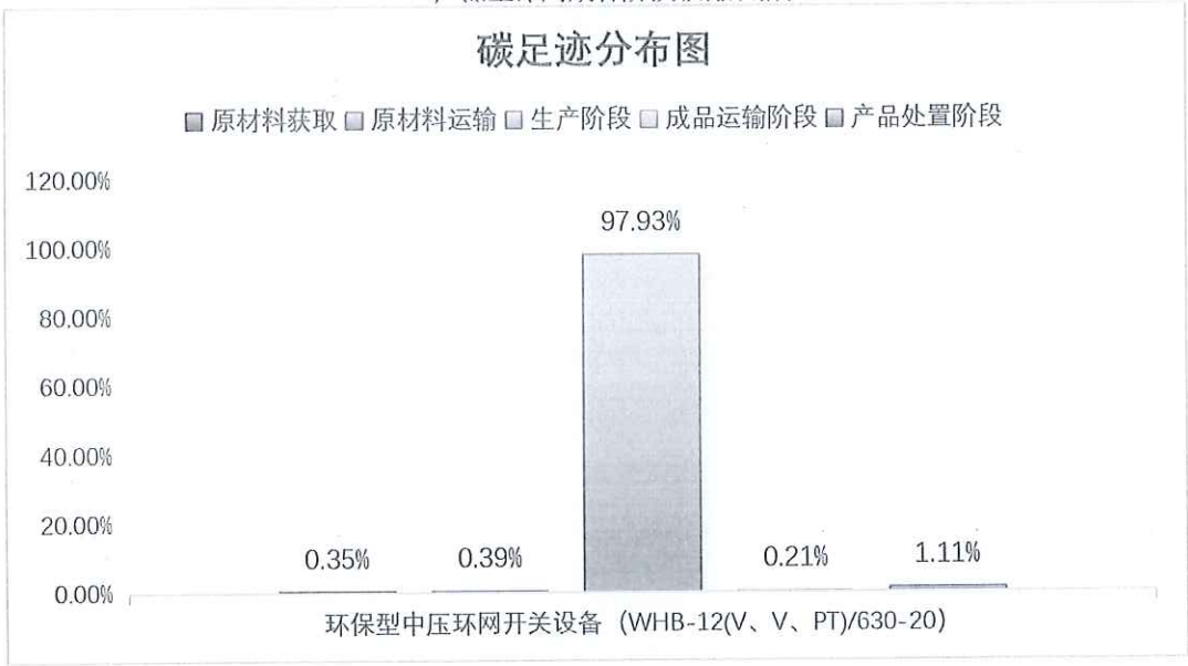
图 5.2-2 1 台环保型中压环网开关设备（WHB-12(V、V、PT)/630-20） 产品生命周期阶段碳排放分布图
