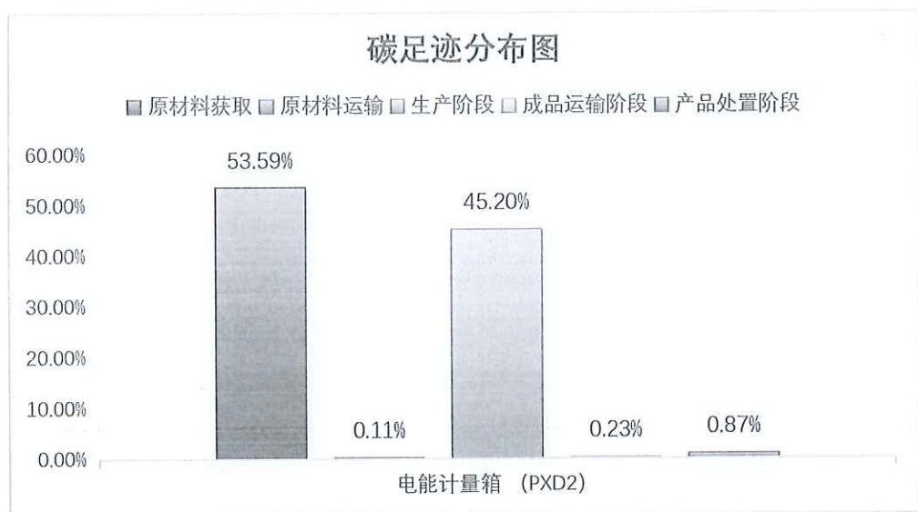
图 5.2-2 1 台电能计量箱（PXD2） 产品生命周期阶段碳排放分布图
