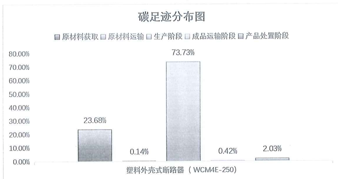
图 5.2-2 1 台塑料外壳式断路器（WCM4E-250） 产品生命周期阶段碳排放分布图
