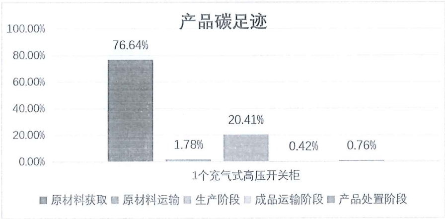
图 5.2-2 1 台充气式高压开关柜（QCS（X）） 产品生命周期阶段碳排放分布图
